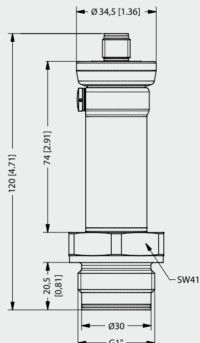
P41 | G1" DIN 3852
