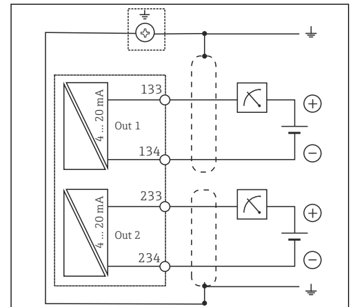
15 Wiring diagram
